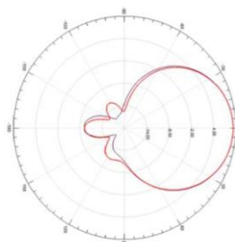
垂直方向图 Elevation
