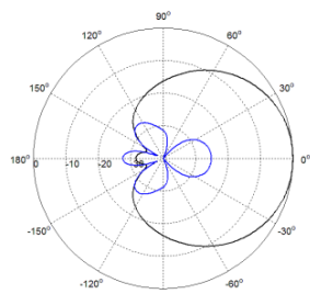
水平方向图 Azimuth
