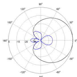
低频水平方向图 Azimuth(Low Band)
