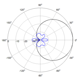
低频垂直方向图 Elevation(Low Band)
