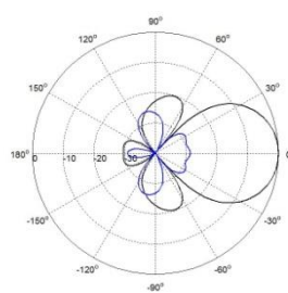
高频水平方向图 Azimuth(High Band)
