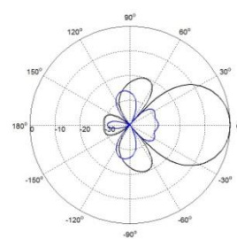
高频垂直方向图 Elevation(High Band)
